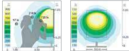
Curvas fotométricas
