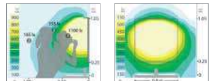
Curvas fotométricas
