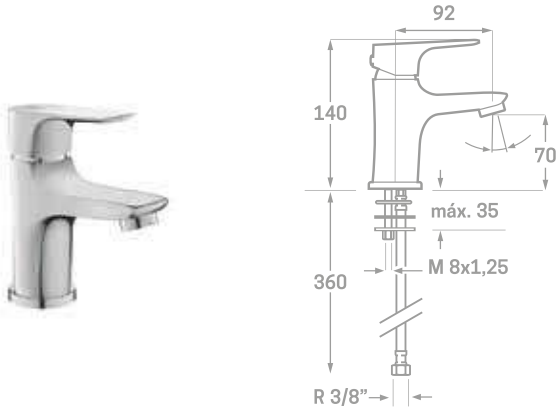
MONOMANDO LAVABO
